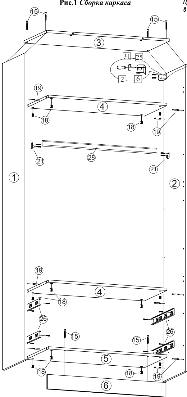
Рис.1 Сборка каркаса
