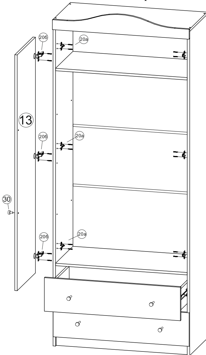
Рис.4 Окончательная сборка
