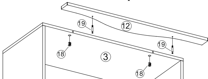
Рис.3 Монтаж Карниза
